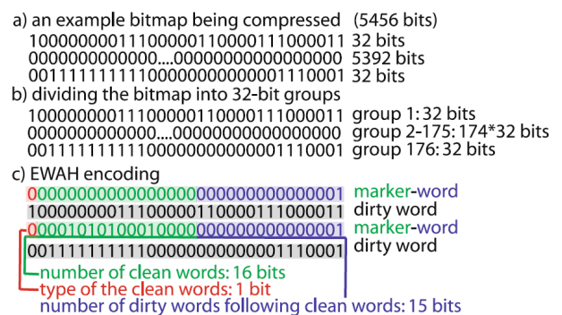
Fig. 5 EWAH encoding method.
