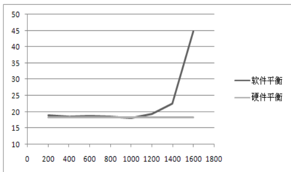
图 13 控制周期测试结果
