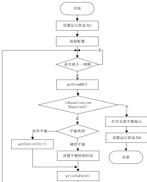
图 7 EQUALIZATION 程序流程
