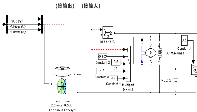
图4 电池单元与充放电控制模型
