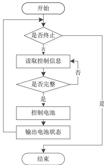
图3 MATLAB 仿真的运行流程
