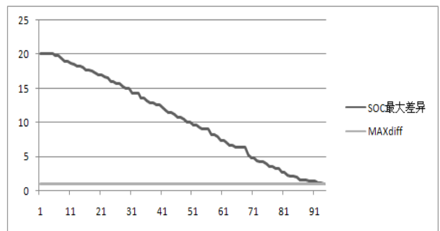
图 12 电池平衡实验结果
