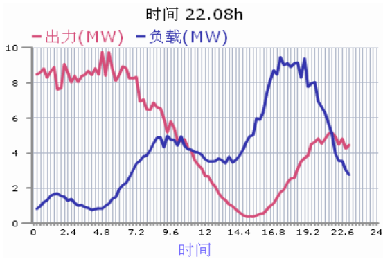
图 10 出力-负载曲线效果图
