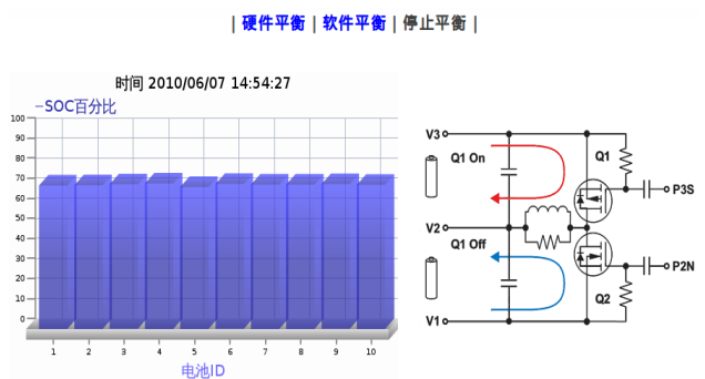
图 9 电池平衡页面效果图
