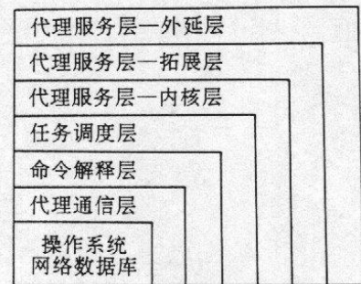
图 4 新一代 CIMS 应用集成平台系统单元结构模型
